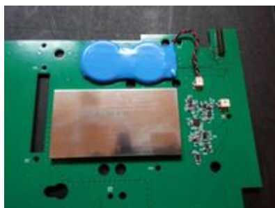
Version modifiée du plus grand circuit imprimé du téléphone (avec dispositif de surveillance). La batterie (en bleu) et le module isolé (en marron clair) font partie du dispositif de surveillance.
