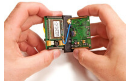
Module d'émission-réception (ouvert)
